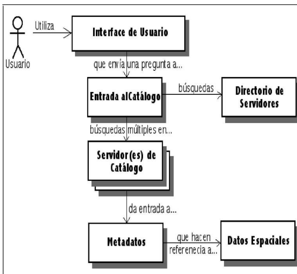
Figura 1: Interacción con servicios de catálogo distribuido
